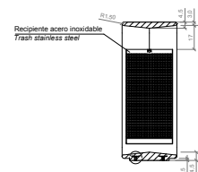
SECCIÓN / SECTION: B-B'
