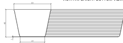
ALZADO / FRONT VIEW ESC. 1:20
